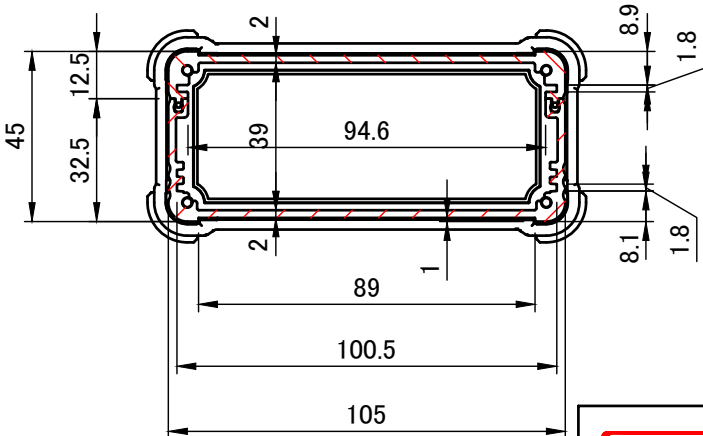
A-A ( 1 : 2 )
