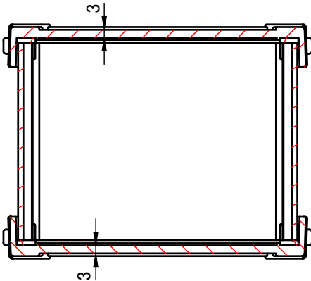
D-D ( 1 : 2 )
