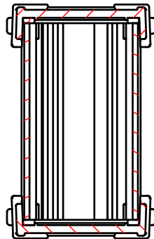
B-B ( 1 : 2 )
