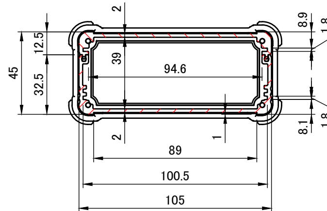
A-A (1:2)
