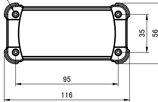
A-A (1:2)
