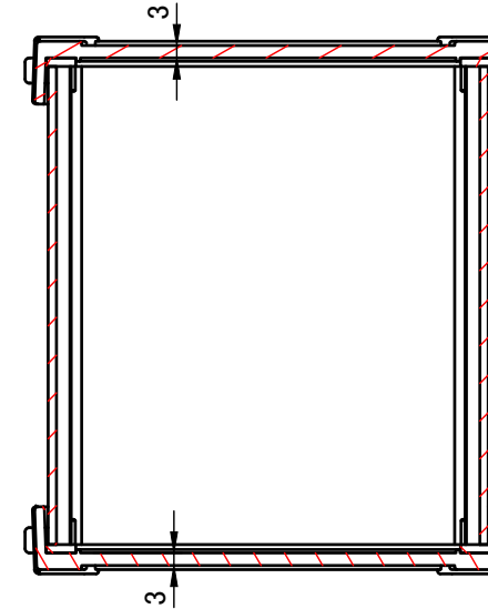
D-D (1:2)
