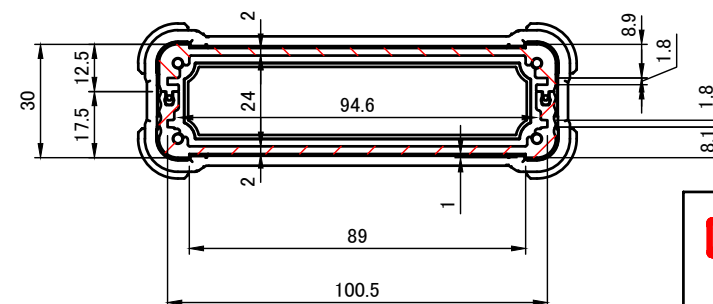
A-A (1:2)
