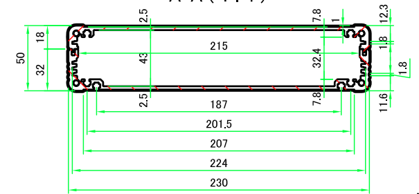
A-A (1:4)
