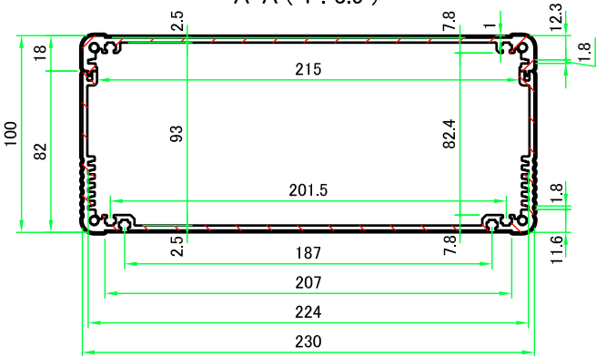
A-A ( 1 : 3.5 )
