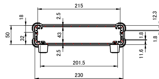
A-A (1:5)
