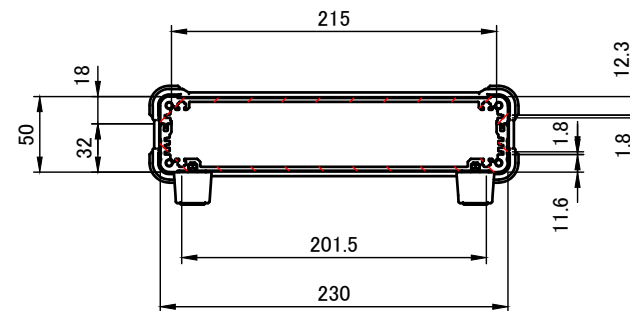
A-A (1:5)
