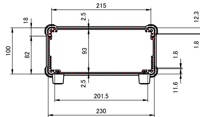
A-A (1:5)
