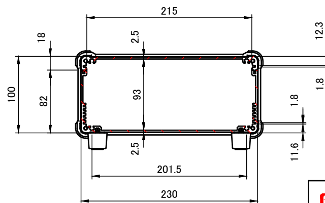
A-A (1:5)
