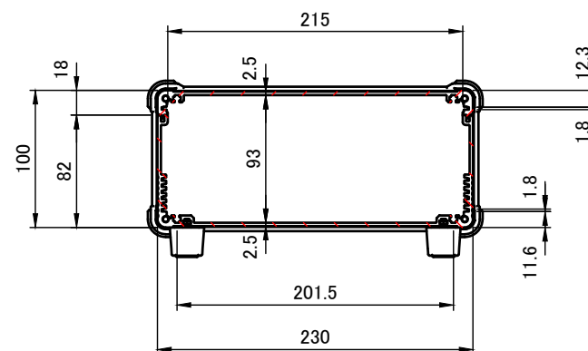
A-A (1:5)
