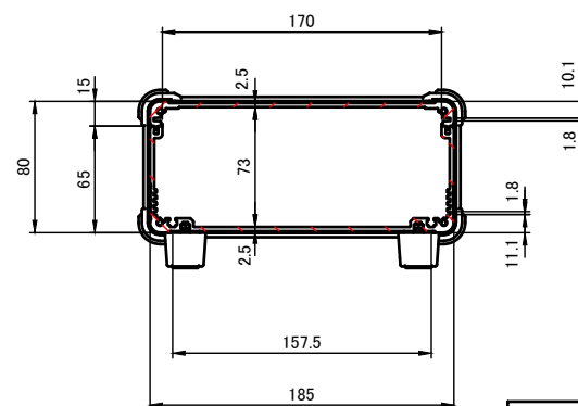
A-A (1:5)
