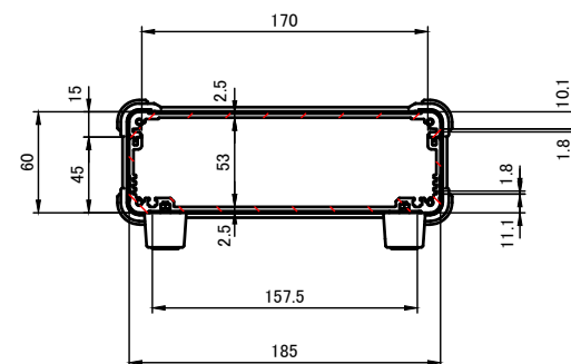
A-A (1:5)
