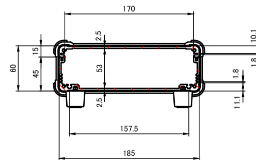
A-A ( 1 : 5 )
