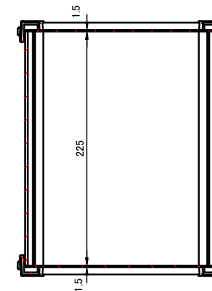
C-C ( 1 : 5 )
