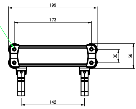
A-A ( 1 : 5 )
