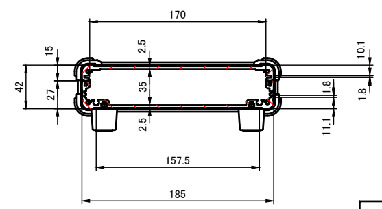
A-A ( 1 : 5 )
