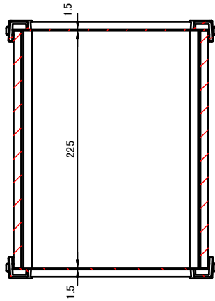
C-C ( 1 : 5 )
