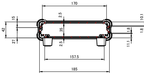
A-A ( 1 : 5 )
