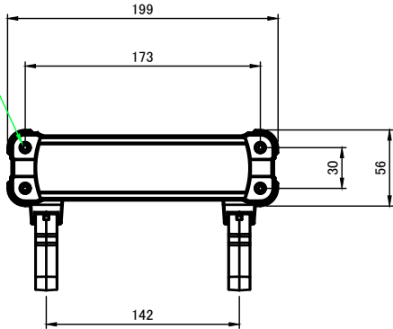
A-A ( 1 : 5 )
