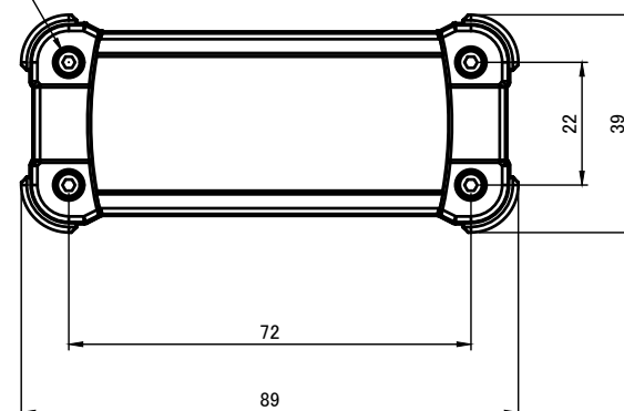
A-A ( 1 : 1.5 )
