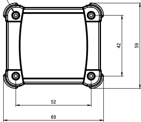
A-A (1:1.5)
