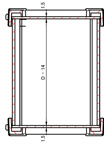
D-D (1:1.5)
