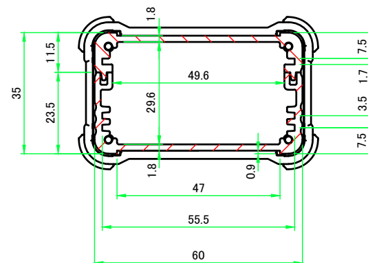
A-A ( 1 : 1.5 )
