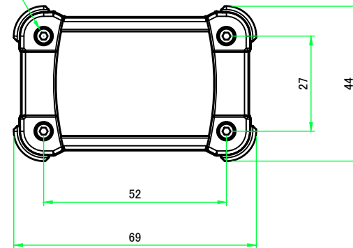
A-A ( 1 : 1.5 )
