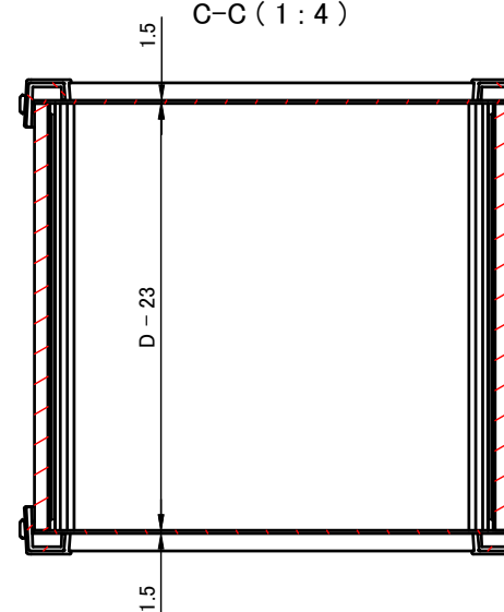
C-C ( 1 : 4 )
