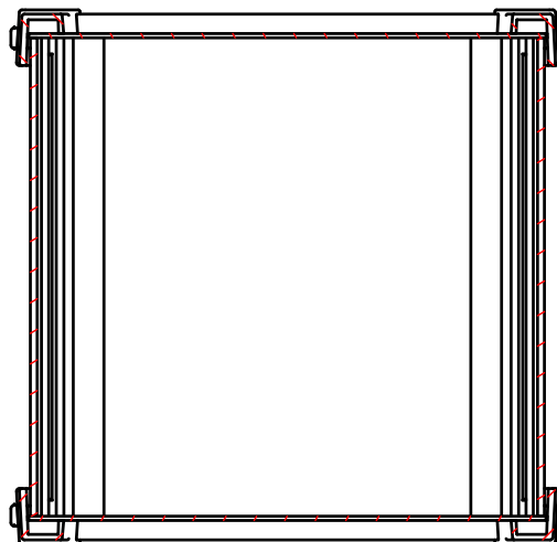
D-D (1:3)
