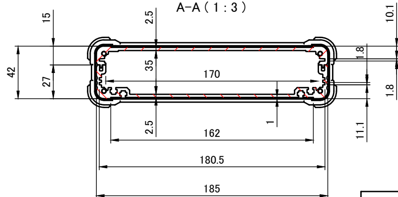
A-A (1:3)
