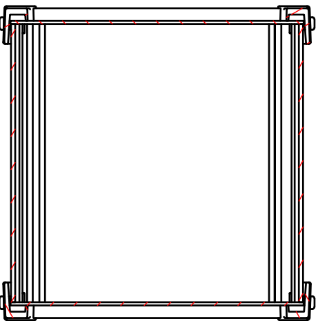
C-C ( 1 : 2.5 )
