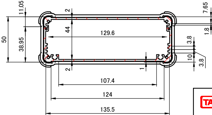
A-A ( 1 : 2.5 )
