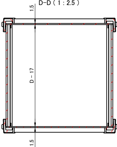
D-D ( 1 : 2.5 )
