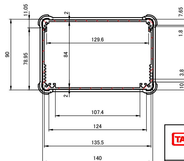
A-A (1:3)
