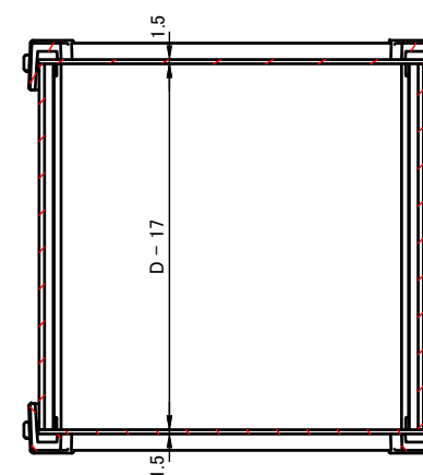
D-D (1:3)
