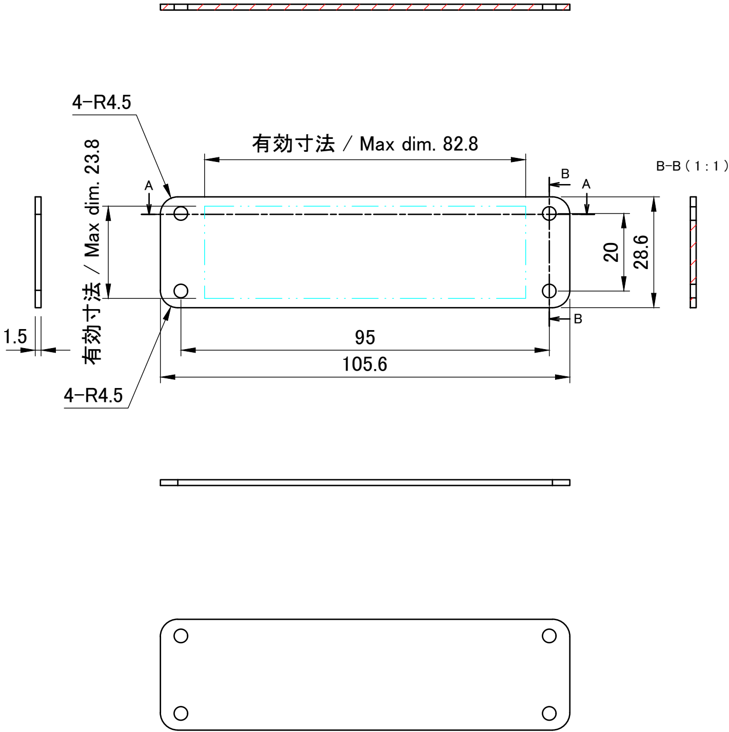
A-A (1:1)
