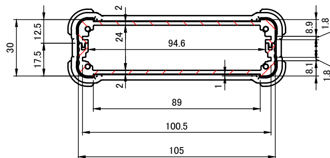
A-A (1:2)
