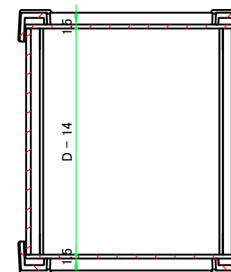
C-C (1:2)
