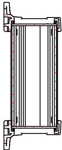
B-B (1:2)
