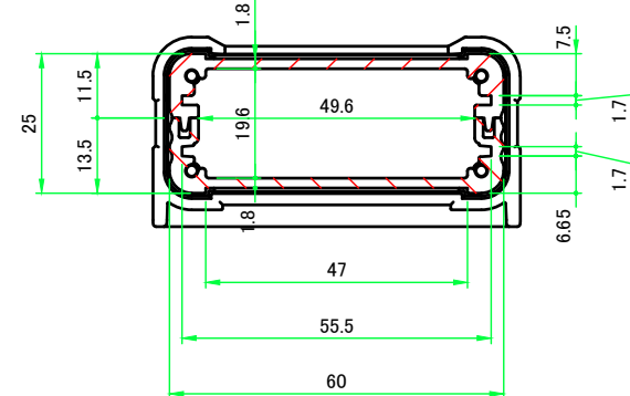
A-A ( 1 : 1.5 )
