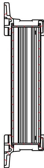
B-B ( 1 : 2.5 )
