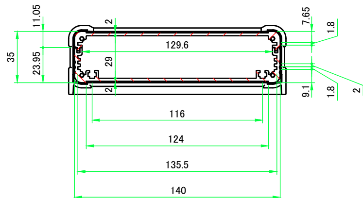
A-A ( 1 : 2.5 )
