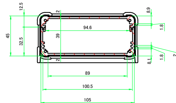
A-A ( 1 : 2.5 )
