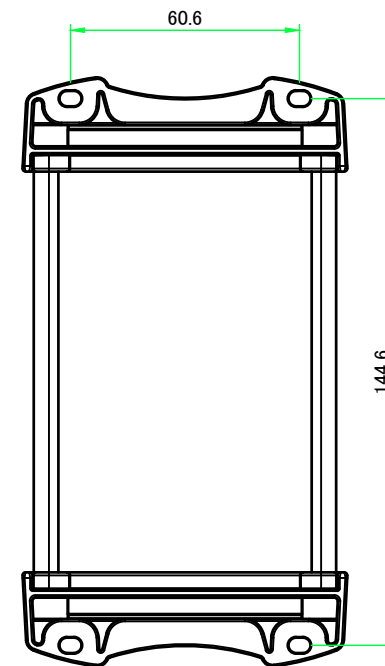
C-C (1:2)
