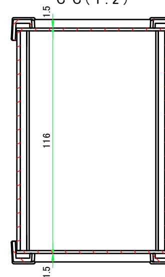
C-C (1:2)
