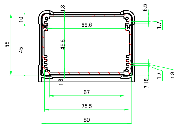
A-A (1:2)
