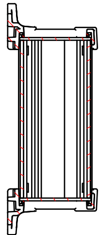
B-B (1:2)
