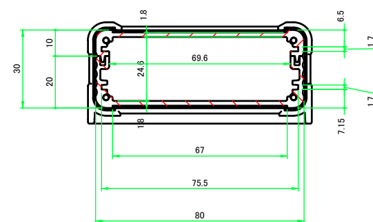
A-A (1:2)
