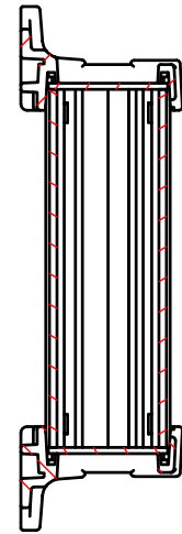
B-B (1:2)
