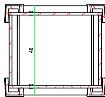
C-C ( 1 : 1.5 )
