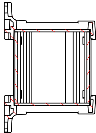
B-B ( 1 : 1.5 )
