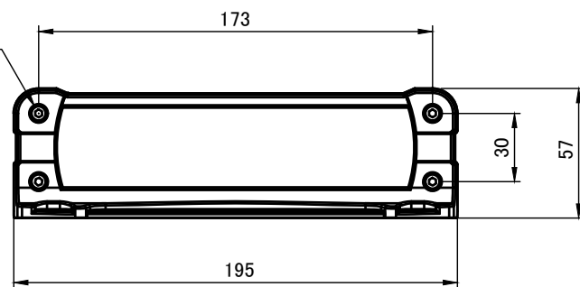
A-A (1:3)
