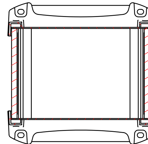
D-D (1:3)
