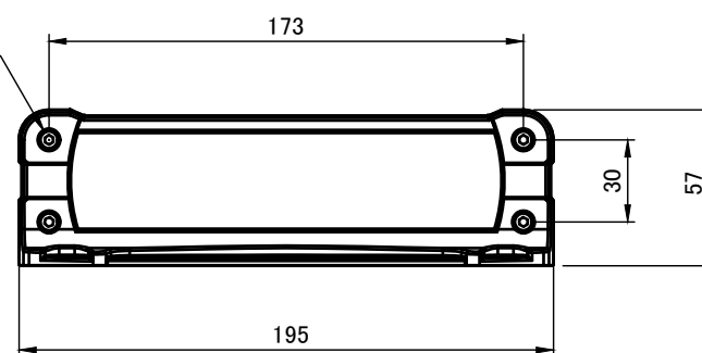
A-A (1:3)
