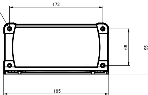
A-A (1:4)
