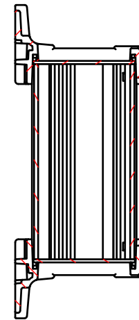
B-B (1:2.5)
