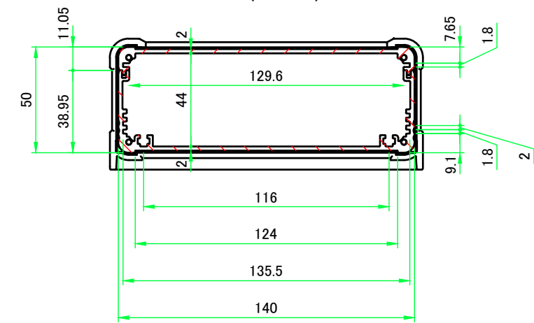
A-A (1:2.5)
