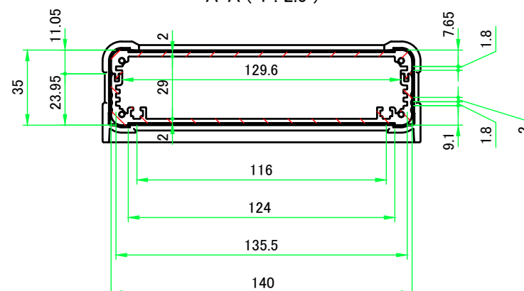
A-A ( 1 : 2.5 )
