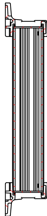
B-B ( 1 : 2.5 )
