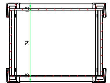
C-C ( 1 : 2.5 )
