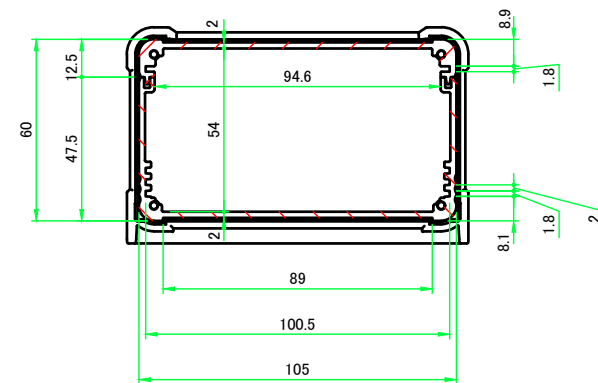
A-A ( 1 : 2.5 )
