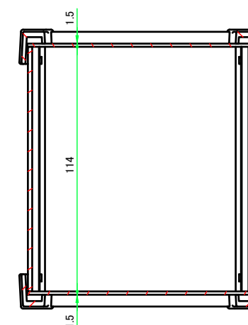
C-C ( 1 : 2.5 )
