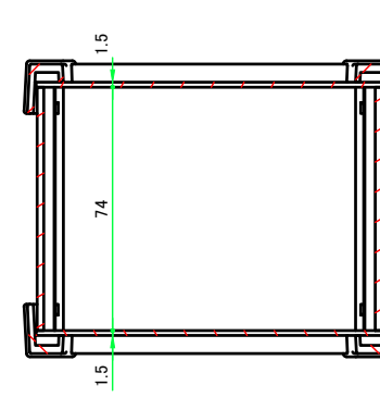
C-C ( 1 : 2.5 )
