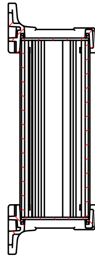
B-B ( 1 : 2.5 )
