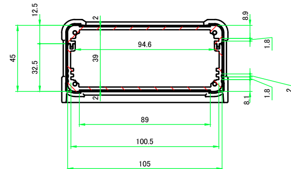
A-A ( 1 : 2.5 )
