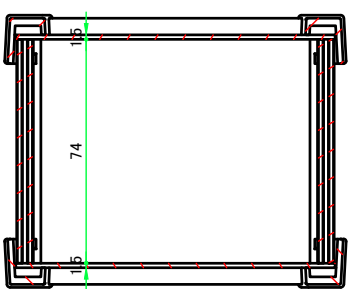
C-C ( 1 : 2.5 )
