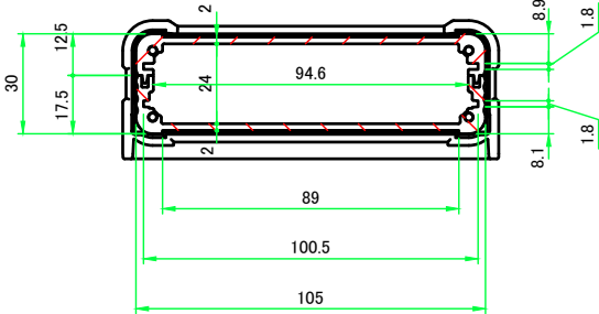
A-A ( 1 : 2.5 )
