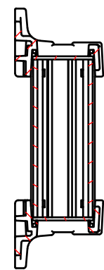
B-B ( 1 : 2.5 )
