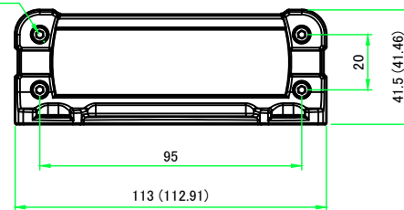
A-A ( 1 : 2.5 )
