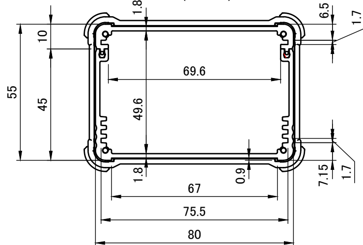
A-A (1:1.5)
