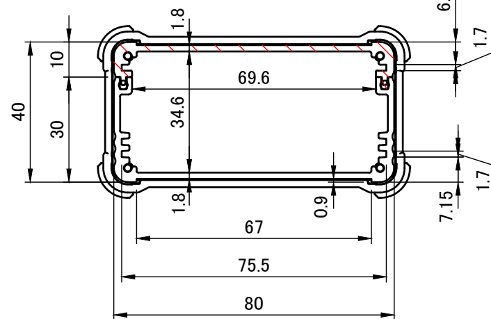
A-A (1:1.5)
