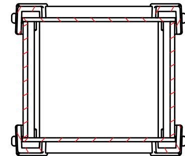
D-D (1:1.5)
