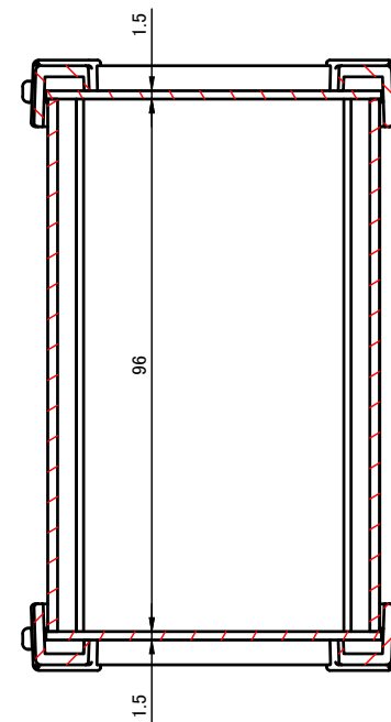
C-C ( 1 : 1.5 )
