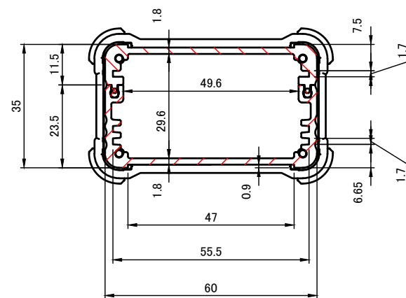
A-A ( 1 : 1.5 )
