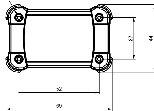
A-A ( 1 : 1.5 )
