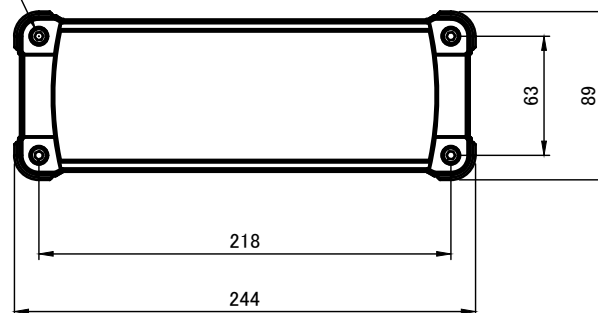
A-A (1:4)
