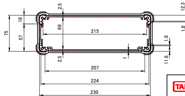
A-A (1:4)
